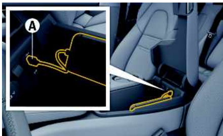
2 pav.: USB sąsaja (C tipo) viduriniame porankyje
