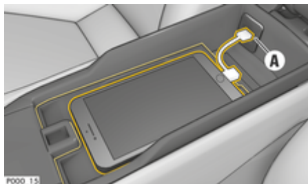
Abb. 2: USB-интерфейс в центральной консоли
