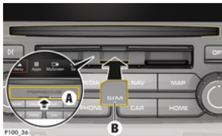
1 pav. Išorinės SIM kortelės įdėjimas ir išėmimas
