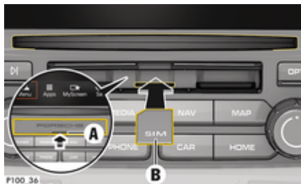
Bild 1: Sätta in och ta ut det externa SIM-kortet
