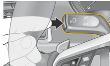
Afb. 12: Spraakbedieningstoets op de hendel
