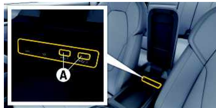
図8：アームレスト内の USB インターフェース (タイプ C)
