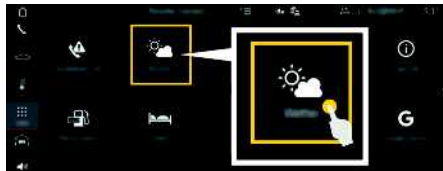
Abb. 15: Wetter
