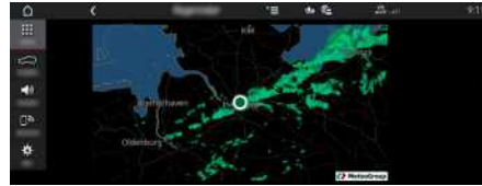
Fig. 10 : Radar des précipitations
