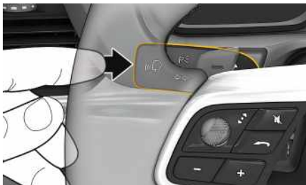
Рис. 3: Кнопка голосового управления на переключателе
