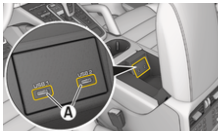
Fig. 3: Interface USB (type C) dans l'accoudoir
