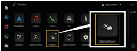
Obr. 16: Počasí
