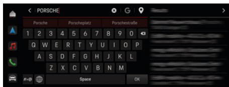
Obr. 7: Vyhledávač
