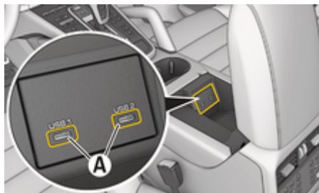
Obr. 1: Rozhraní USB (typ C) v loketní opěrce
