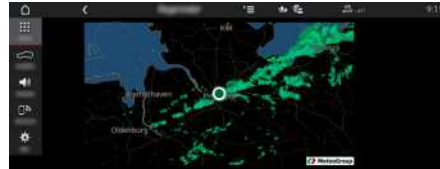
Fig. 21: Rain Radar
