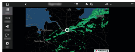
Rys. 15: Radar deszczu
