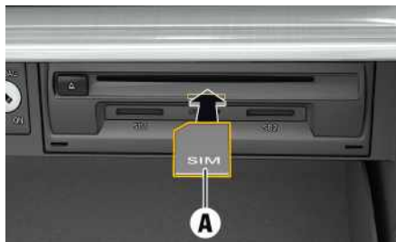
Рис. 1: Установка и извлечение внешней SIM-карты в перчаточном ящике
