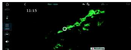
図 14: 雨レーダー
