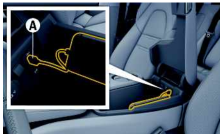
Kuva 2: Keskiäksinojan USB-liitäntä (tyyppi C)
