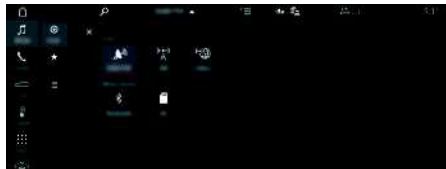
Рис. 15: Radio Plus
