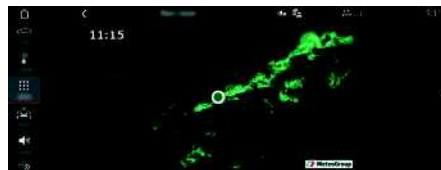
Рис. 9: Радар дождя
