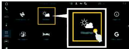
Рис. 8: Погода
