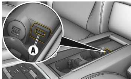
Fig. 3: Interfaccia USB nella consolle centrale della zona posteriore
