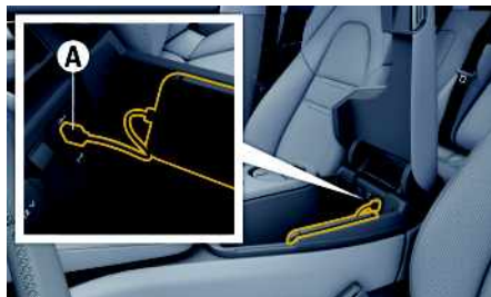
Rys. 3: Port USB (typu C) w podłokietniku środkowym
