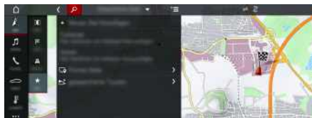
Bild 11: Öppna portalmål
