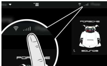
Bild 10: Öppna enhetshanteraren
